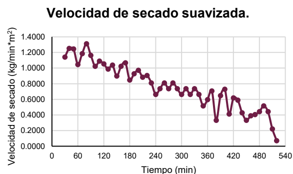
Figura 14. Velocidad de secado suavizada a través del tiempo de operación.
